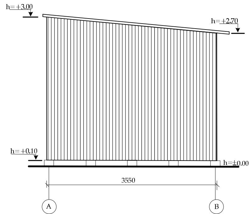
Fasādes skice pa asīm A-B M=1:100
