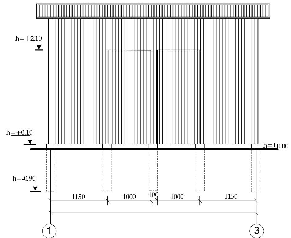
Fasādes skice pa asīm 1-3 M=1:100
