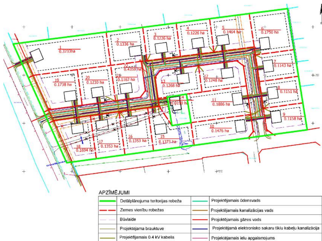
Attēls Nr. 10. Inženiertīklu shēma. Inženiertīklu risinājumus skatīt Grafiskās daļas plānā Nr. 3 “Inženiertīklu plāns”
