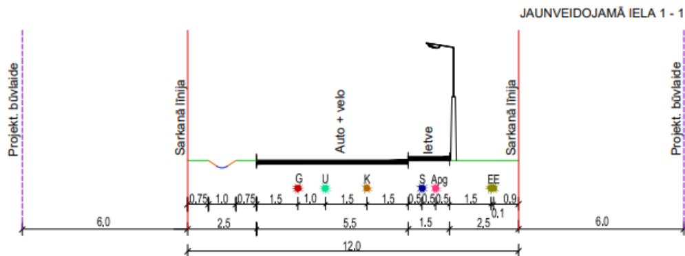
Attēls Nr. 8. Jaunveidojamās ielas šķērsprofils 1-1.
