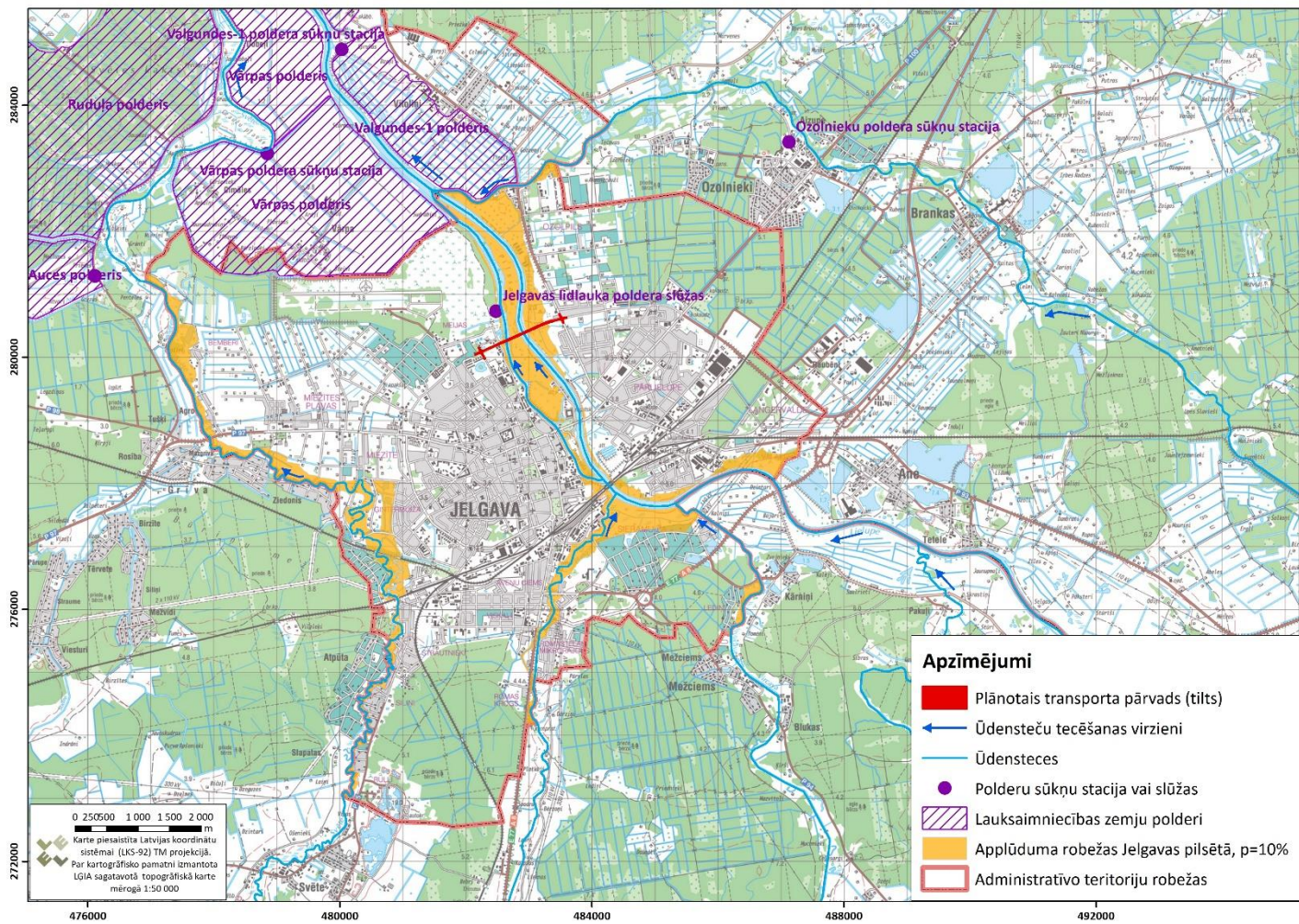
3. attēls. Paredzētās darbības teritorijai tuvāko ūdensteču un Jelgavas pilsētas applūduma robežu pārskata plāns (pavasara palu ar atkārtotās varbūtību p=10\% situācijai)
