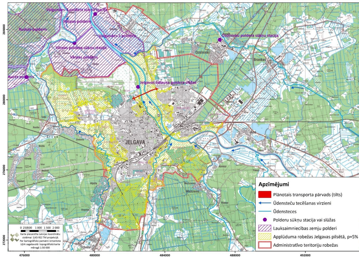
2. attēls. Paredzētās darbības teritorijai tuvāko ūdensteču un Jelgavas pilsētas applūsuma robežu pārskata plāns (pavasara palu ar atkārtotās varbūtību p= 5% situācijai)
