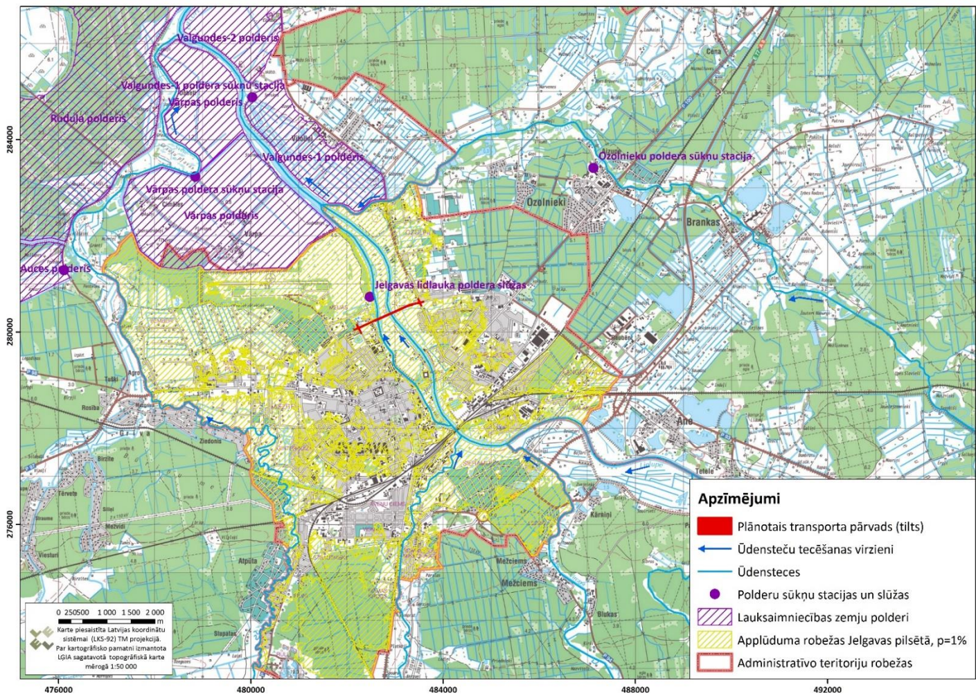
1. attēls. Paredzētās darbības teritorijai tuvāko ūdensteču un Jelgavas pilsētas applūsuma robežu pārskata plāns (pavasara palu ar atkārtotās varbūtību p= 1% situācijai)
