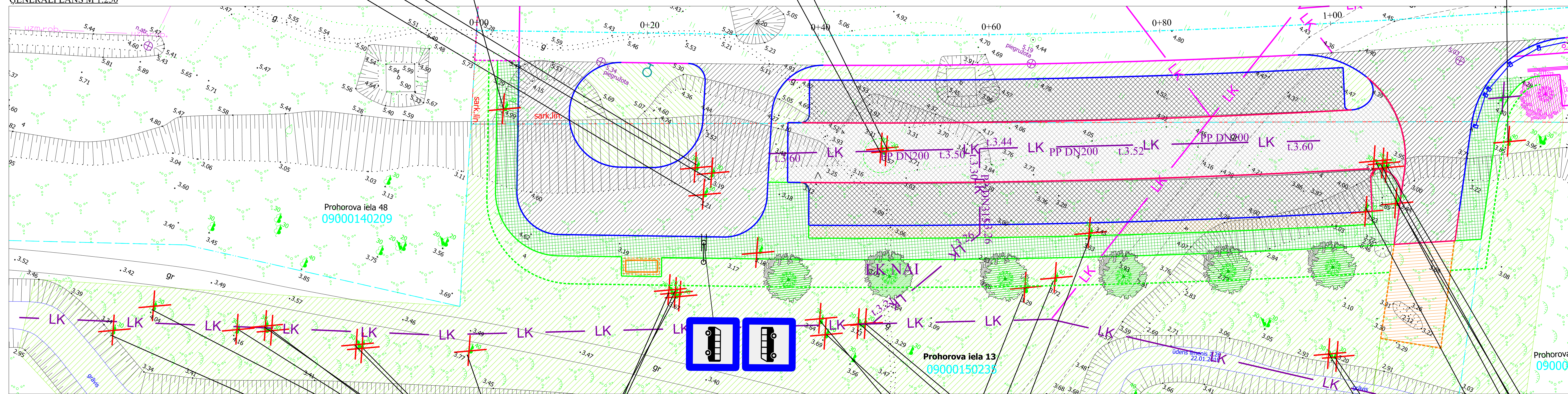
GENERĀLPLĀNS M 1:250
